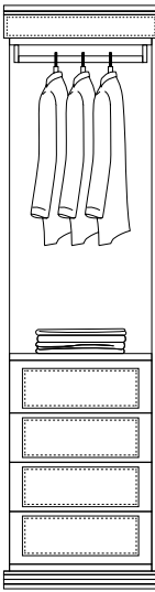
SN107 senza anta SNV107 anta vetro SNL107 anta legno CM 60 X 60 X 235,5 H
