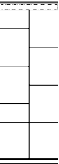
SB001-CX CM 84,5 X 4,5 X 235,5 H
