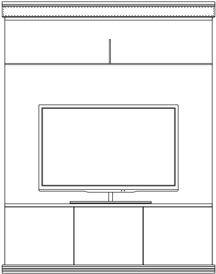
S011 senza anta CM 180 X 46 X 235,5 H
