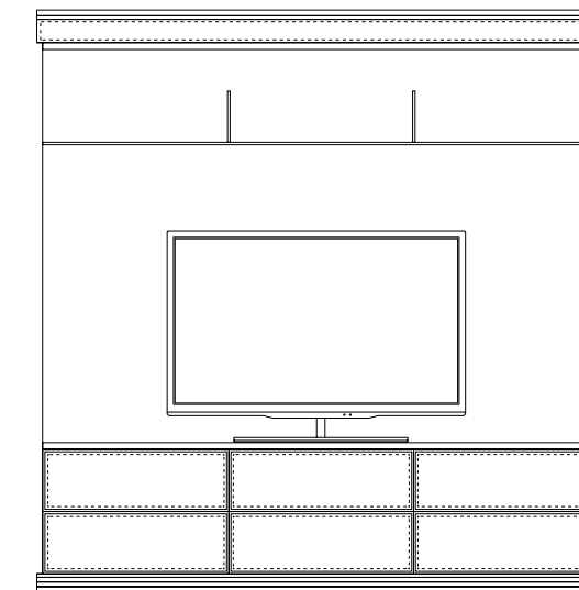
S009 senza anta CM 225 X 46 X 235,5 H
