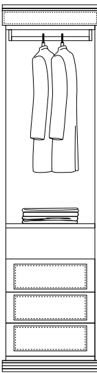
SN108 senza anta SNV108 anta vetro SNL108 anta legno CM 60 X 60 X 235,5 H
