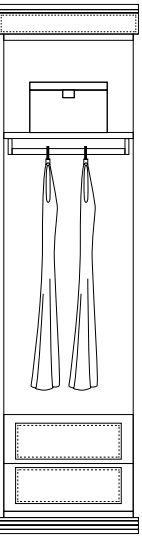
SN104 senza anta SNV104 anta vetro SNL104 anta legno CM 60 X 60 X 235,5 H
